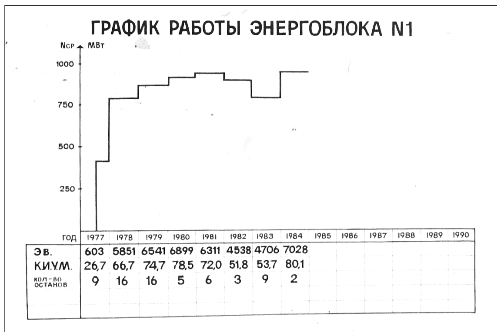
Графік роботи енергоблока № 1 за 1977-1984 рр.
