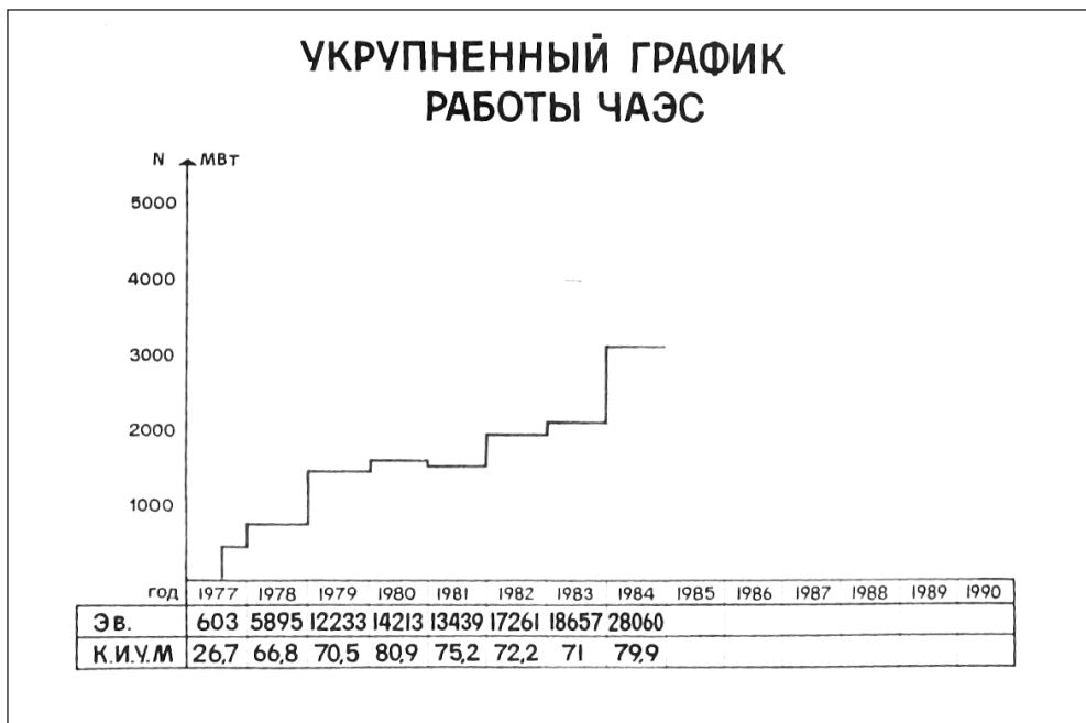
Графік роботи ЧАЕС за 1977–1984 рр. ГДА СБУ. — Ф. 11. — Спр. 991. — Т. 2.
