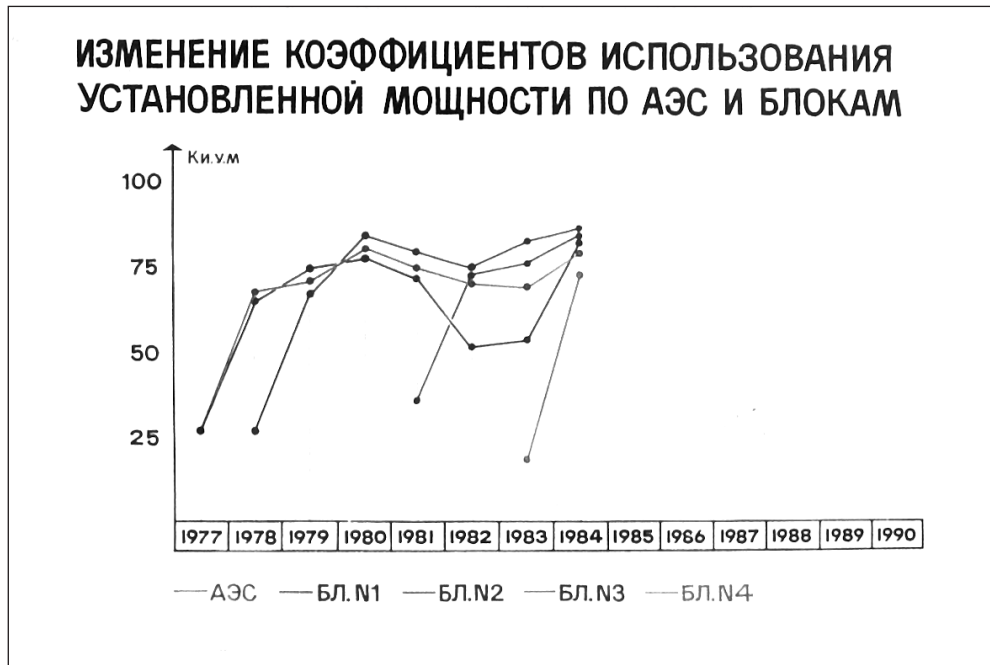
Графік зміни коефіцієнтів використання встановленої потужності енергоблоків ЧАЕС за 1977-1984 рр. ГДА СБУ. — Ф. 11. — Спр. 991. — Т. 2.
