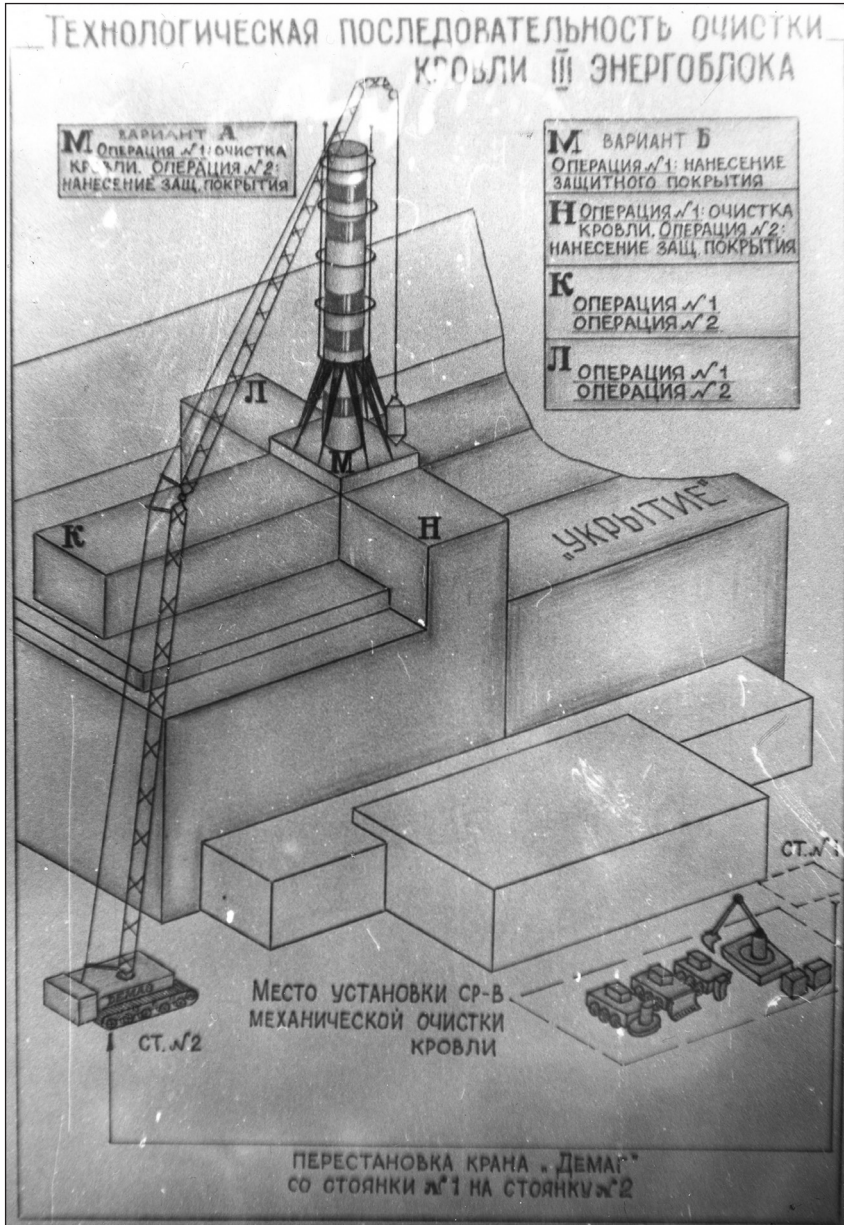
Зображення технологічної послідовності робіт з очищення даху 3 енергблока ЧАЕС. З архіву А.В. Морєва.
