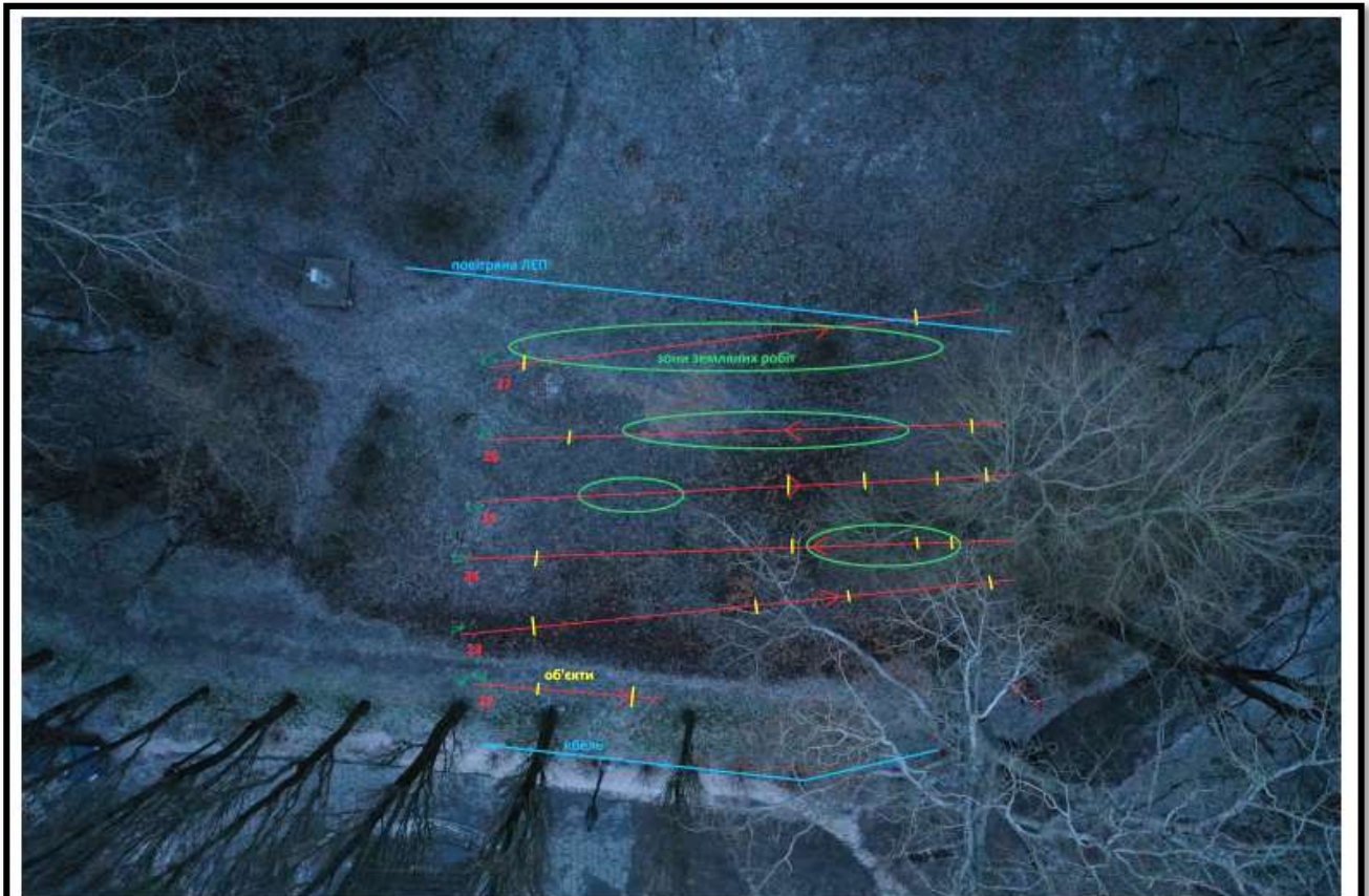
Малюнок 4. Ділянка дослідження георадаром та трасошукачем
