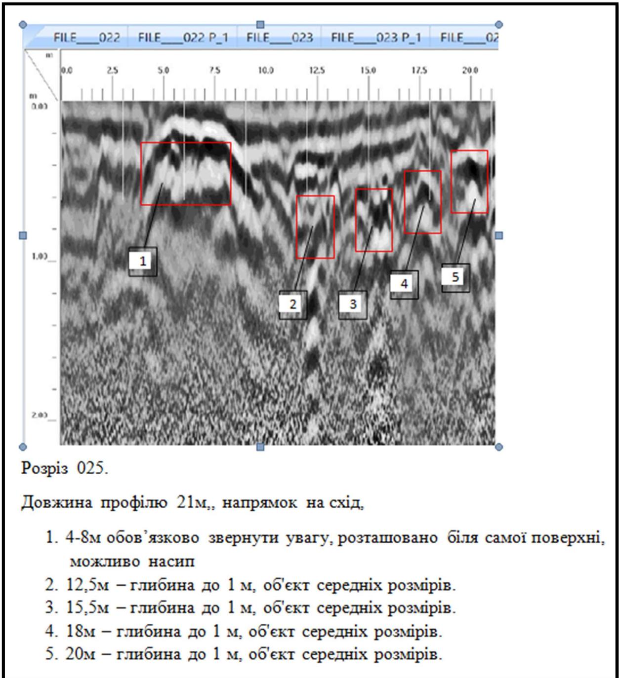
Малюнок № 3. Схема виявлених аномалій згідно «Пояснювальної записки щодо проведених георадарних та трасопошукових вишукувань спрямованих на пошук геологічних аномалій по об'єкту "Заповідник Бабин Яр"» за адресою : м. Київ, вул. Ілленка 46А" за авторством Прокопчука А.Є.
